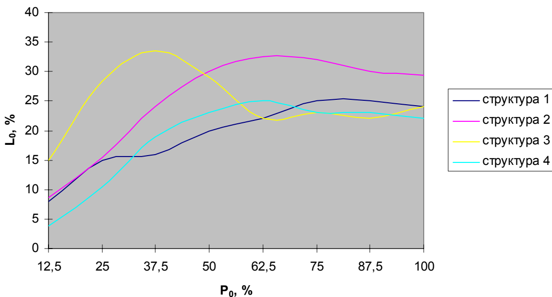
Зависимость относительного изменения интенсивности свечения ( L_0 ) при изменении плотности газа ( P_0 )
